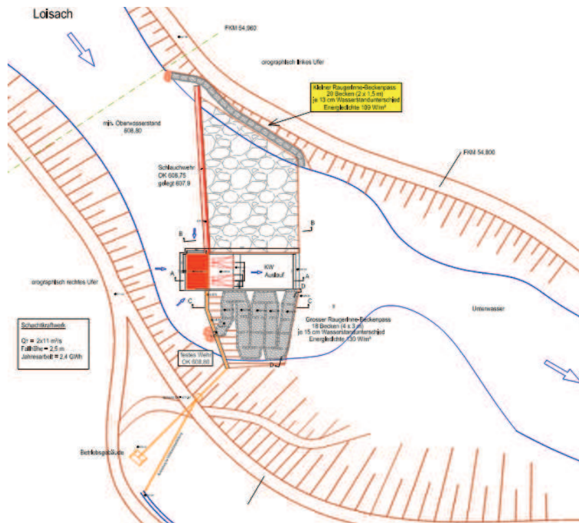
Abbildung 2: Grundkonzept Schachtkraftwerk an der Loisach
